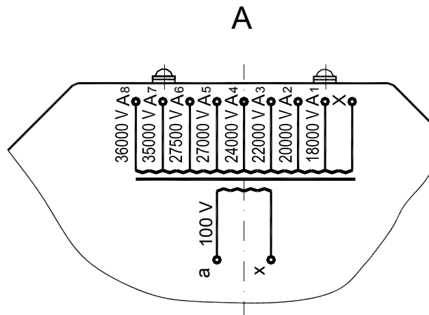
Рисунок А.11 Габаритные, присоединительные размеры и масса трансформаторов напряжения НЛЛ-35-5 (остальное см. рисунок А.6).
