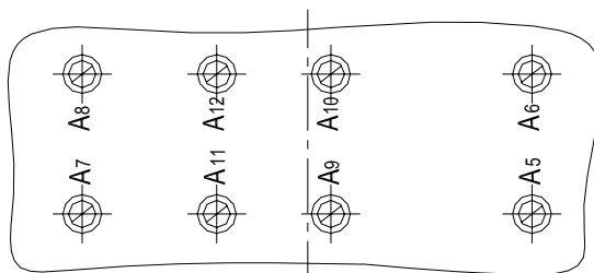
Расположение клемм у трансформаторов напряжения НЛЛ-35, НЛЛ-35-1, НЛЛ-35-2, НЛЛ-35-3, НЛЛ-35-4, НЛЛ-35-5
