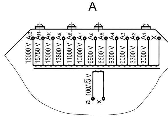
Рисунок А.2. Габаритные, присоединительные размеры и масса трансформаторов напряжения НЛЛ-15-1 (остальное см. рисунок А.1).
