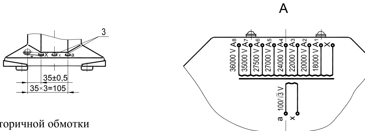
Рисунок А.10 Габаритные, присоединительные размеры и масса трансформаторов напряжения НЛЛ-35-4 (остальное см. рисунок А.6).
