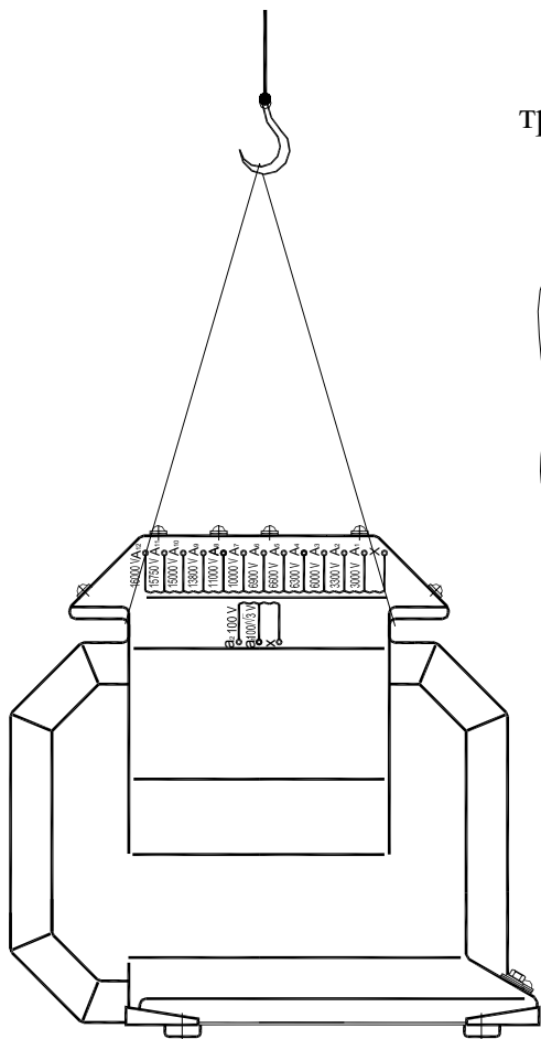
Рисунок Б.1 Способ строповки №1
