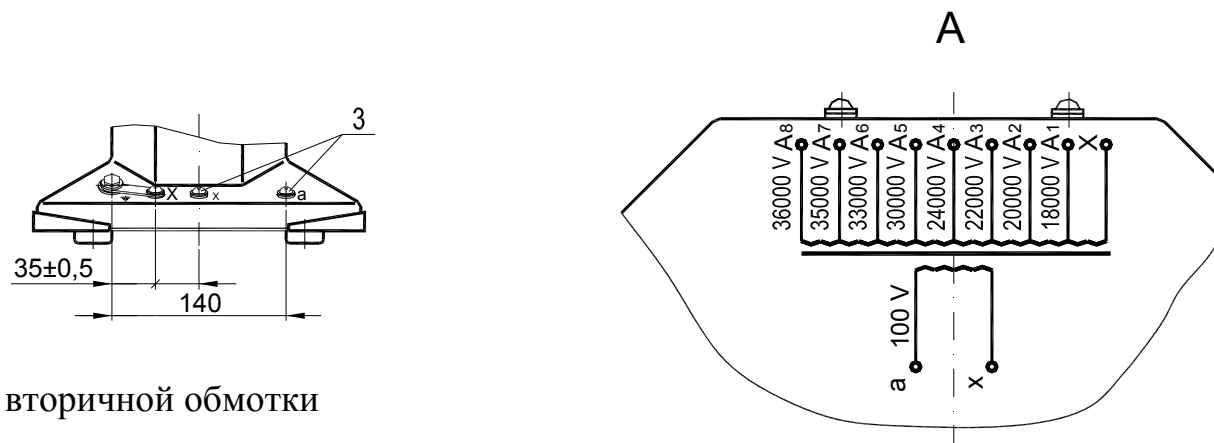
Рисунок А.9 Габаритные, присоединительные размеры и масса трансформаторов напряжения НЛЛ-35-3 (остальное см. рисунок А.6).
