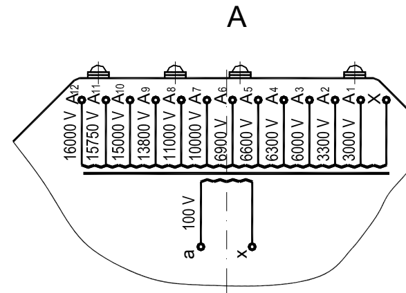
Рисунок А.3. Габаритные, присоединительные размеры и масса трансформаторов напряжения НЛЛ-15-2 (остальное см. рисунок А.1).
