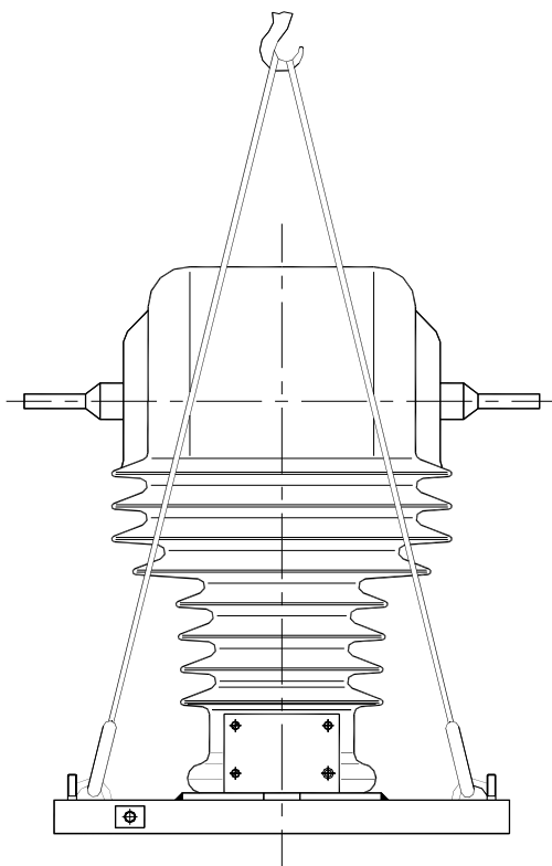
Рисунок В.2 - Схема строповки трансформаторов без рамы
