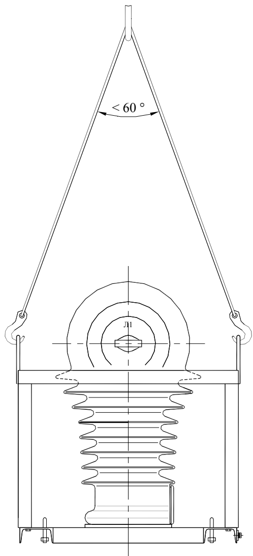
Рисунок В.1 - Схема строповки трансформаторов в раме
