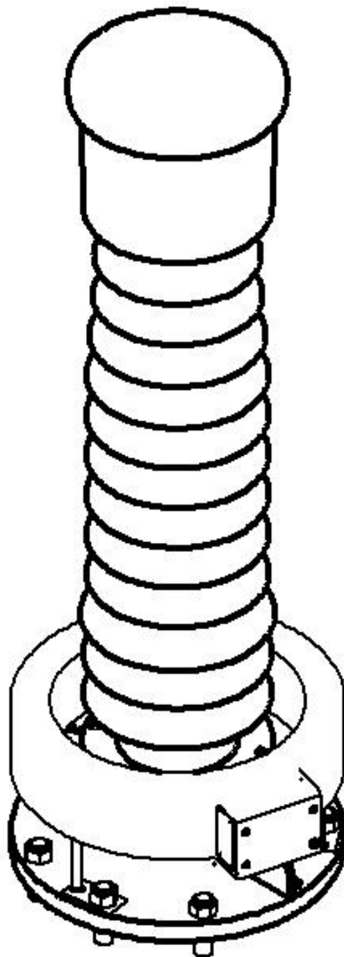
Приложение Г (обязательное) Трансформатор тока ТВ-110-IX на высоковольтном вводе
