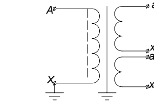
Рисунок А.2 Принципиальная электрическая схема трансформаторов ЗНОЛ.06
