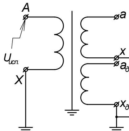
Рисунок В.3 Схема испытания электрической прочности изоляции первичной обмотки трансформатора приложенным напряжением 1,3 номинального частоты 50 Гц
