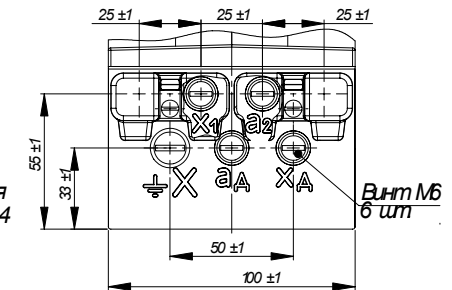
Рисунок А.5 Клеммник для исполнения ЗНОЛ.06.4 (остальное см рисунок А.1)
