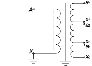
Рисунок А.3 Принципиальная электрическая схема для исполнений ЗНОЛ.06.4
