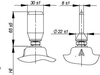
Рисунок А.4 Исполнение высоковольтного ввода трансформаторов для токопроводов (остальное см рисунок А.1)
