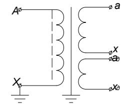
Рисунок Б2 Принципиальная электрическая схема трансформаторов
