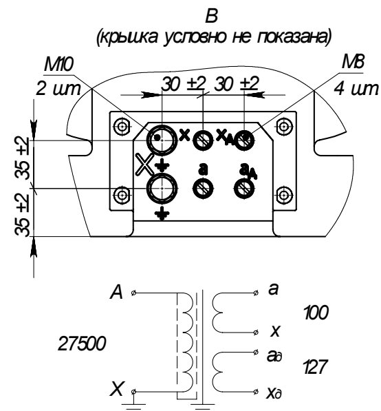
Рисунок А2 Принципиальная электрическая схема трансформаторов на номинальное напряжение первичной обмотки 27500 В
