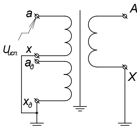
Рисунок Б.2 Схема испытания электрической прочности изоляции первичной обмотки трансформатора индуктированным напряжением при частоте 400 Гц
