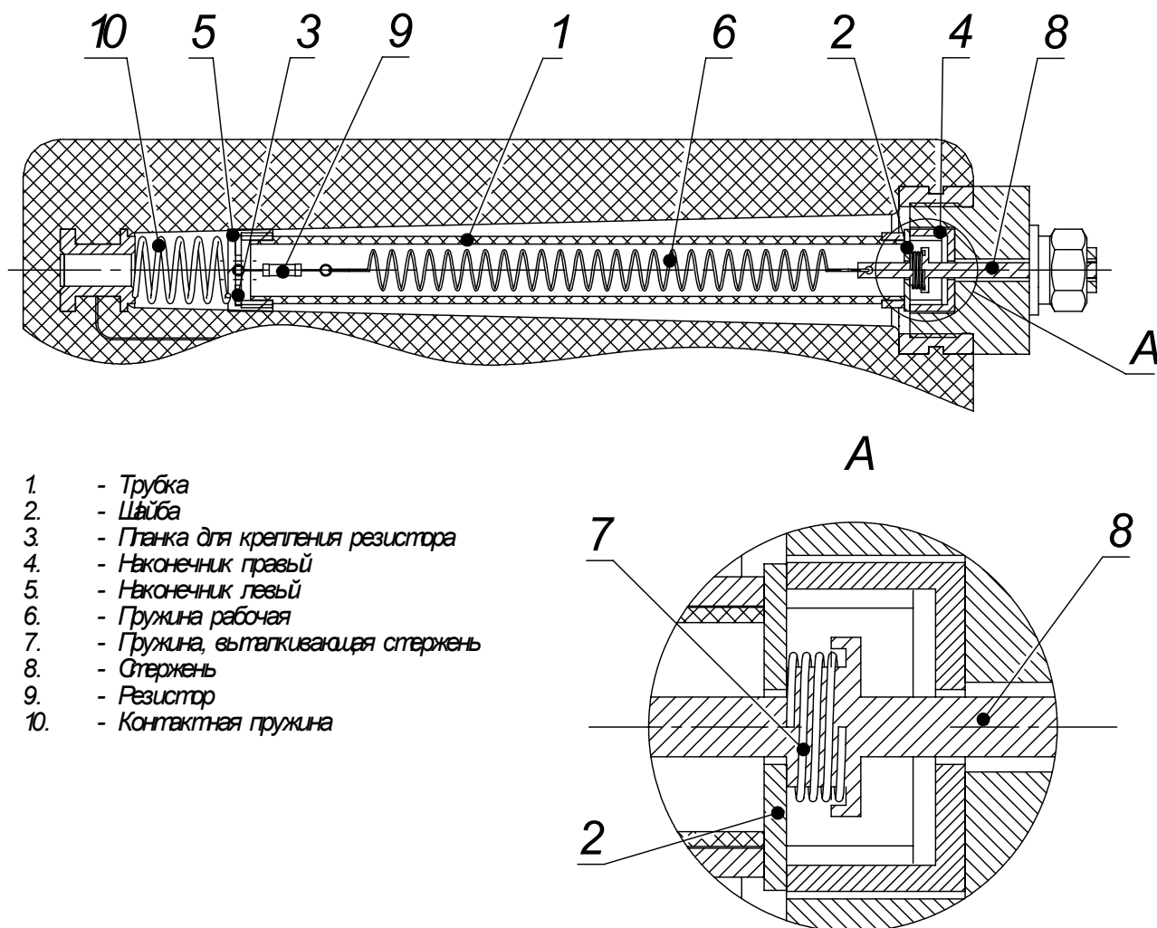
Рисунок В.1 Установка защитного предохранительного устройства в трансформатор ЗНТП
